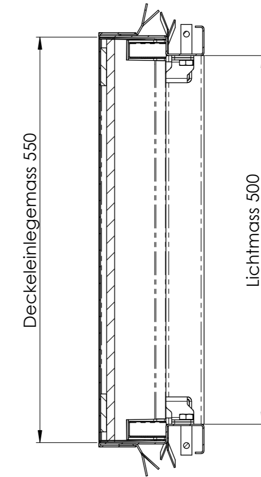
SCHNITT B-B MABSTAB 1 : 5
